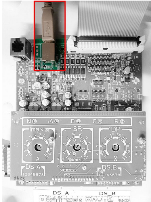
الشكل 6-موصل "USB" في لوحة "EBox" وفي جهاز "Box DConnect"
