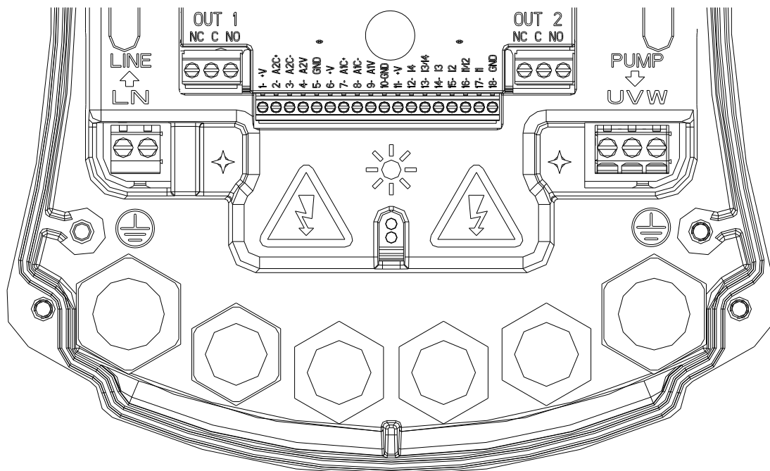
Figura 1: Conexiones eléctricas
