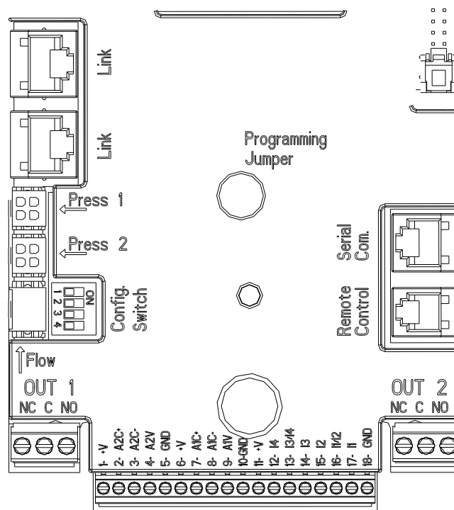
Фиг. 3: Свързвания
