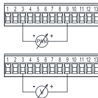
8 pav. Ištraukiama 13 kontaktų gnybtų dėžutė. Įvadais 0-10V ir PWM
