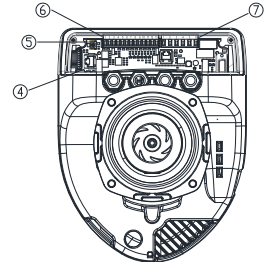
Resim 5: Elektrik bağlantıları (arka)
