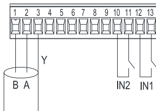
Εικόνα 7: Αφαιρούμενη κλέμια 13 πόλων: ψηφιακές εισοδοι και MODBUS
