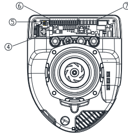
Fig. 5: Elanslutning (baksida)
