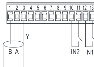
Figur 7: Udtagelig 13-polet klemliste: digitale indgange og MODBUS
